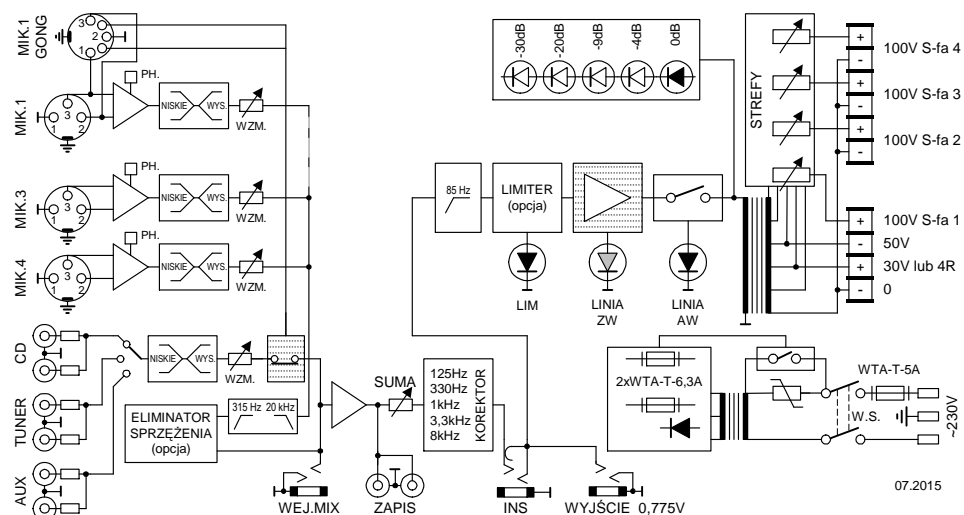
SCHEMAT BLOKOWY WZMACNIACZA MOCY WM-5257
